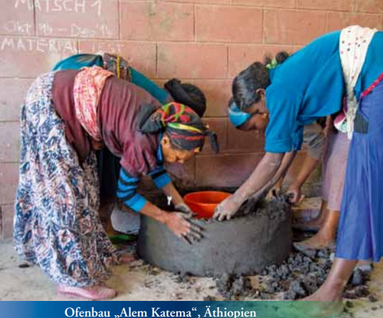
Ofenbau „Alema Katema“, Äthiopien
